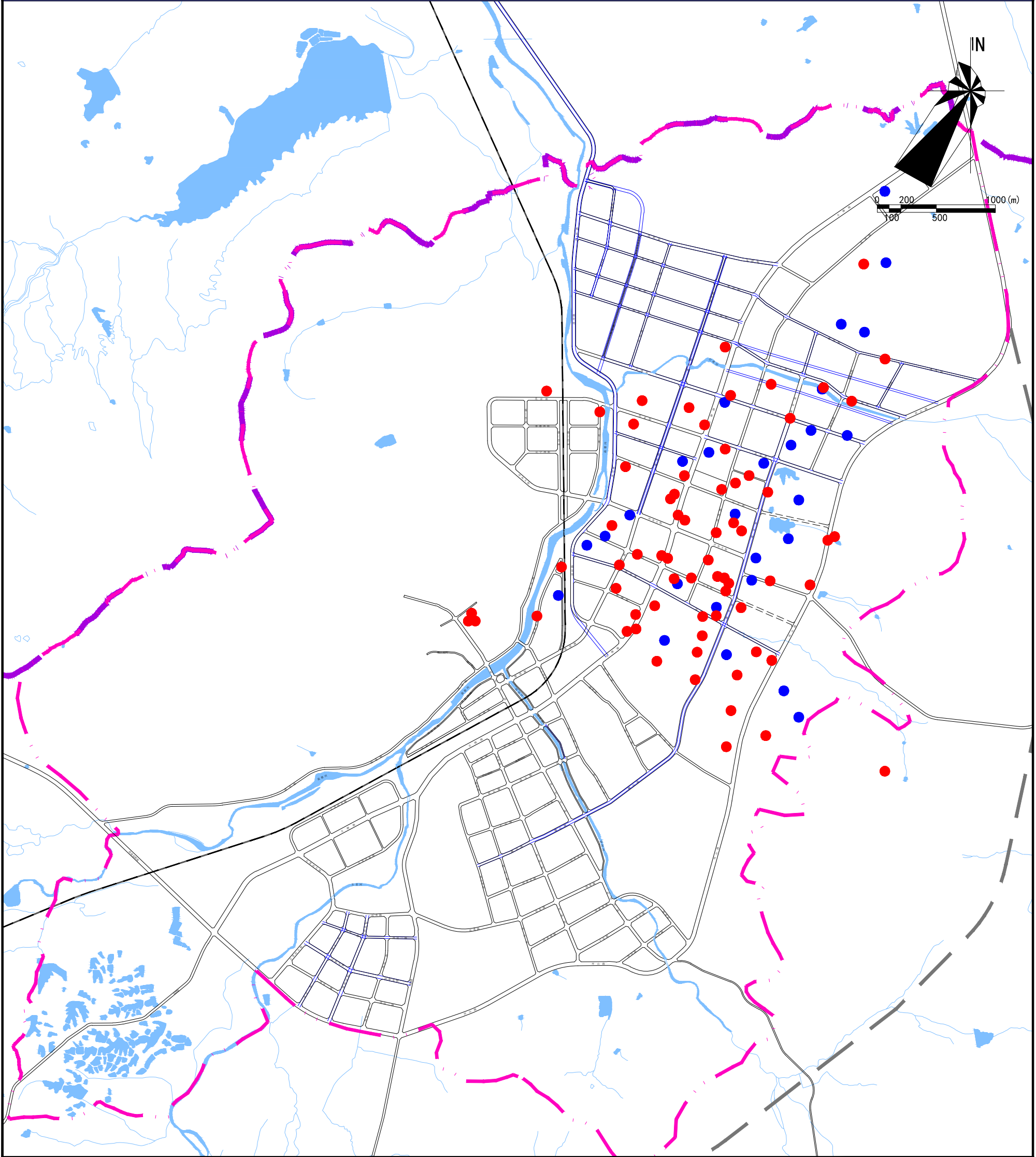
——永吉县中心城区移动通信基站规划图
